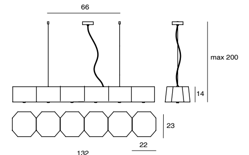
Zhe Pendant P6 SQ-2322MPL6 E27 6 x Max 46W Black textile wire
