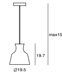
Salute Pendant Cake SQ-828P E27 1 x Max 46W Black textile wire
