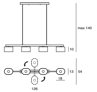
Kazoku Pendant SG-323CTR4 G9 4 x Max 33W Rotatable cross bar Black textile wire
