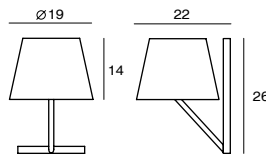
Concom Wall SQ-513MW E14 1 x Max 25W
