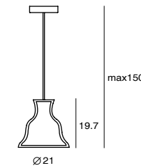
Salute Pendant Bell R SQ-827PR E27 1 x Max 46W Black textile wire
