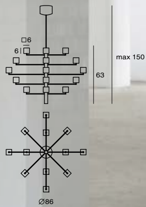
Ice Pendant P20 SD-62CFL20 G4 20 x Max 10W Clear wire
