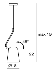
Dodo Pendant SQ-218PS E27 1 x Max 46W Shade rotatable Black textile wire
