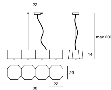
Zhe Pendant P4 SQ-2322MPL4 E27 4 x Max 46W Black textile wire
