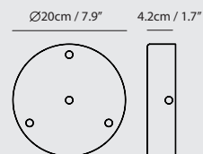
Bracket A14
