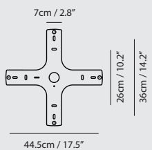
Bracket A17
