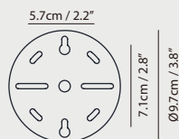
Bracket A3
