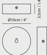
Bracket A3
