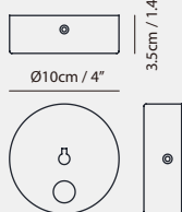
Bracket A4
