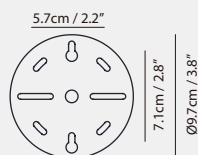
Bracket A4
