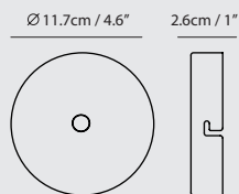
Bracket A8
